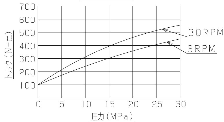
トルク性能表
